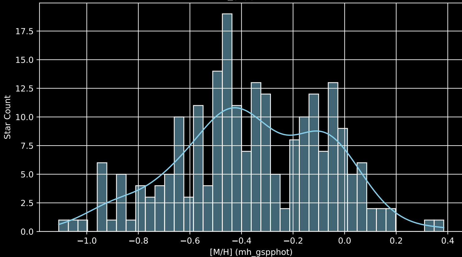
GALAH DR4 Field: [548] [M/H] (mh_gspphot) (n= 221)
