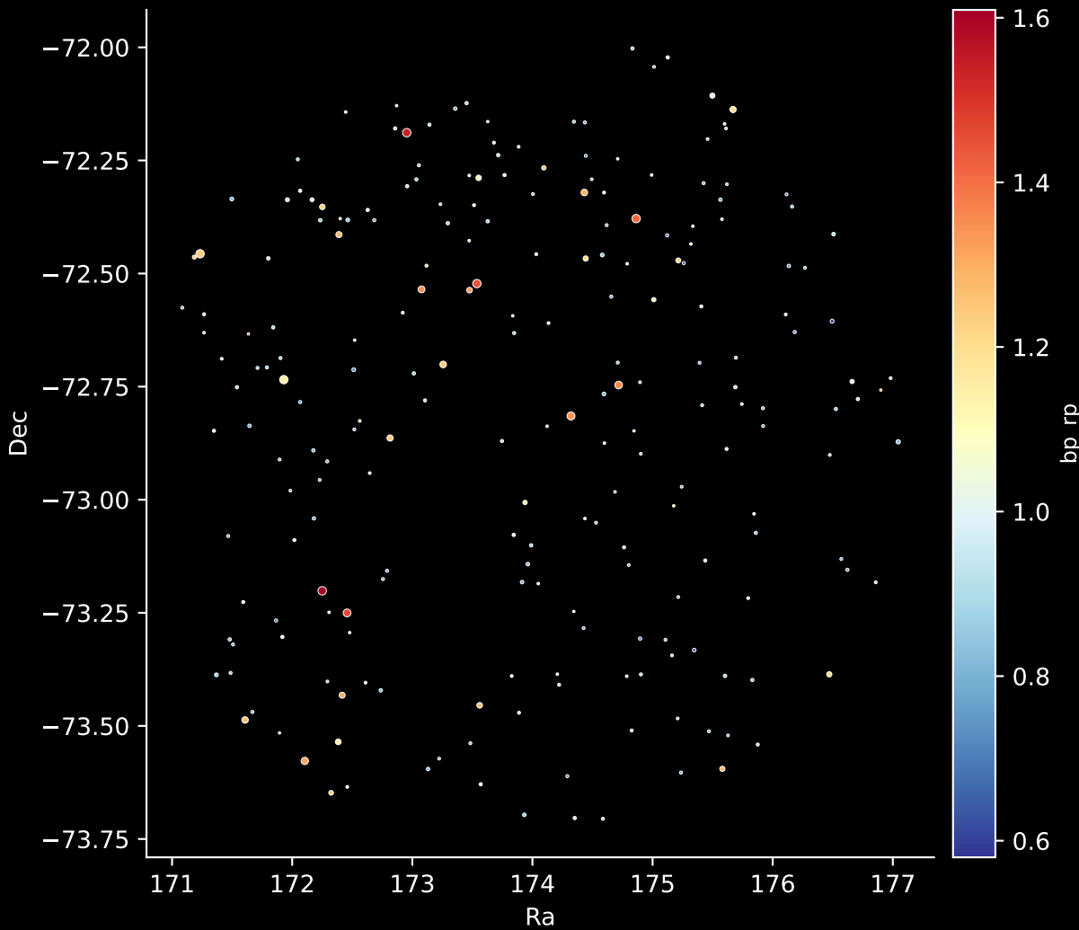
GALAH DR4 Field: [548] Stars: 221
