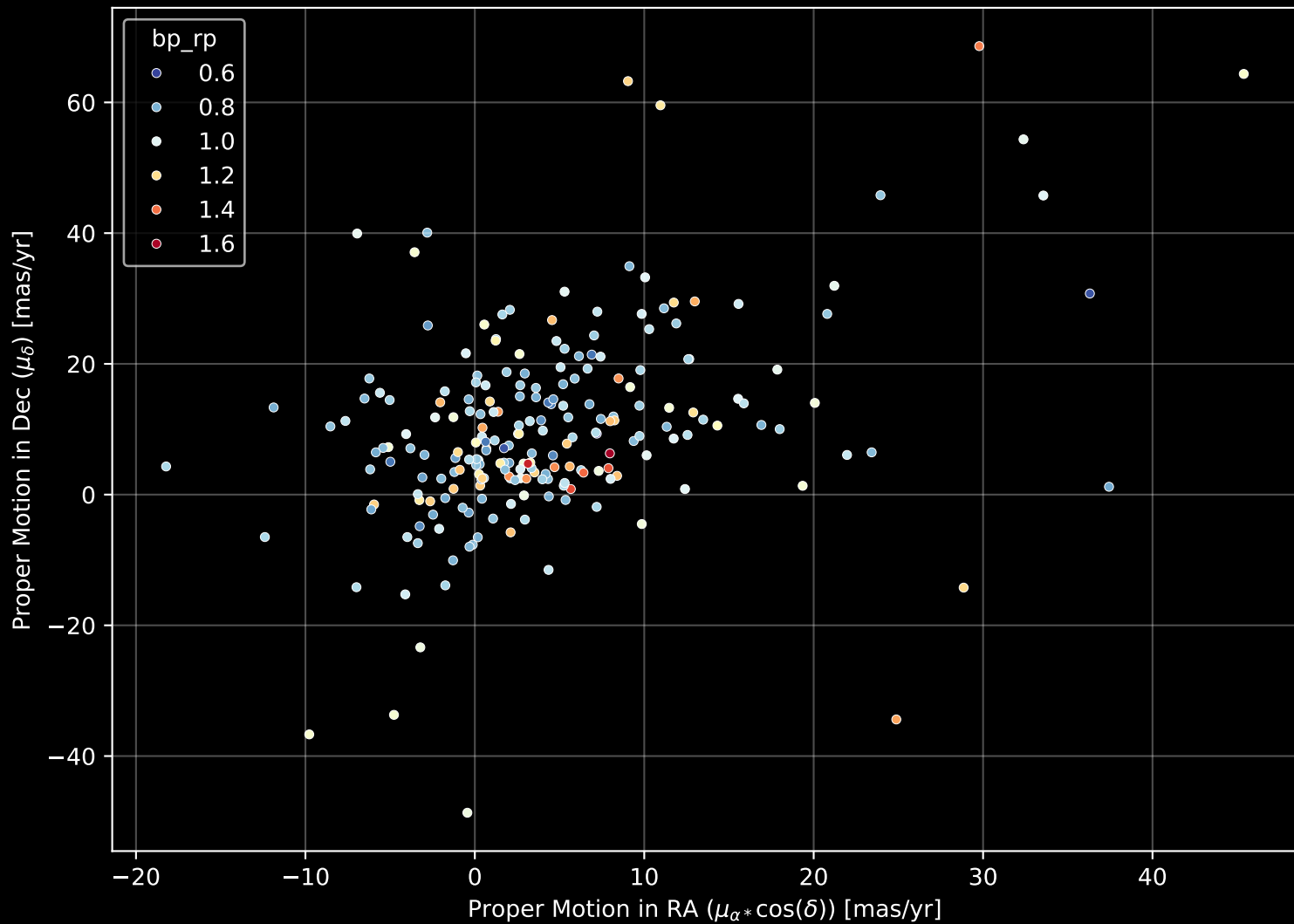
GALAH DR4 Field: [548] Proper Motion Diagram (n= 221)
