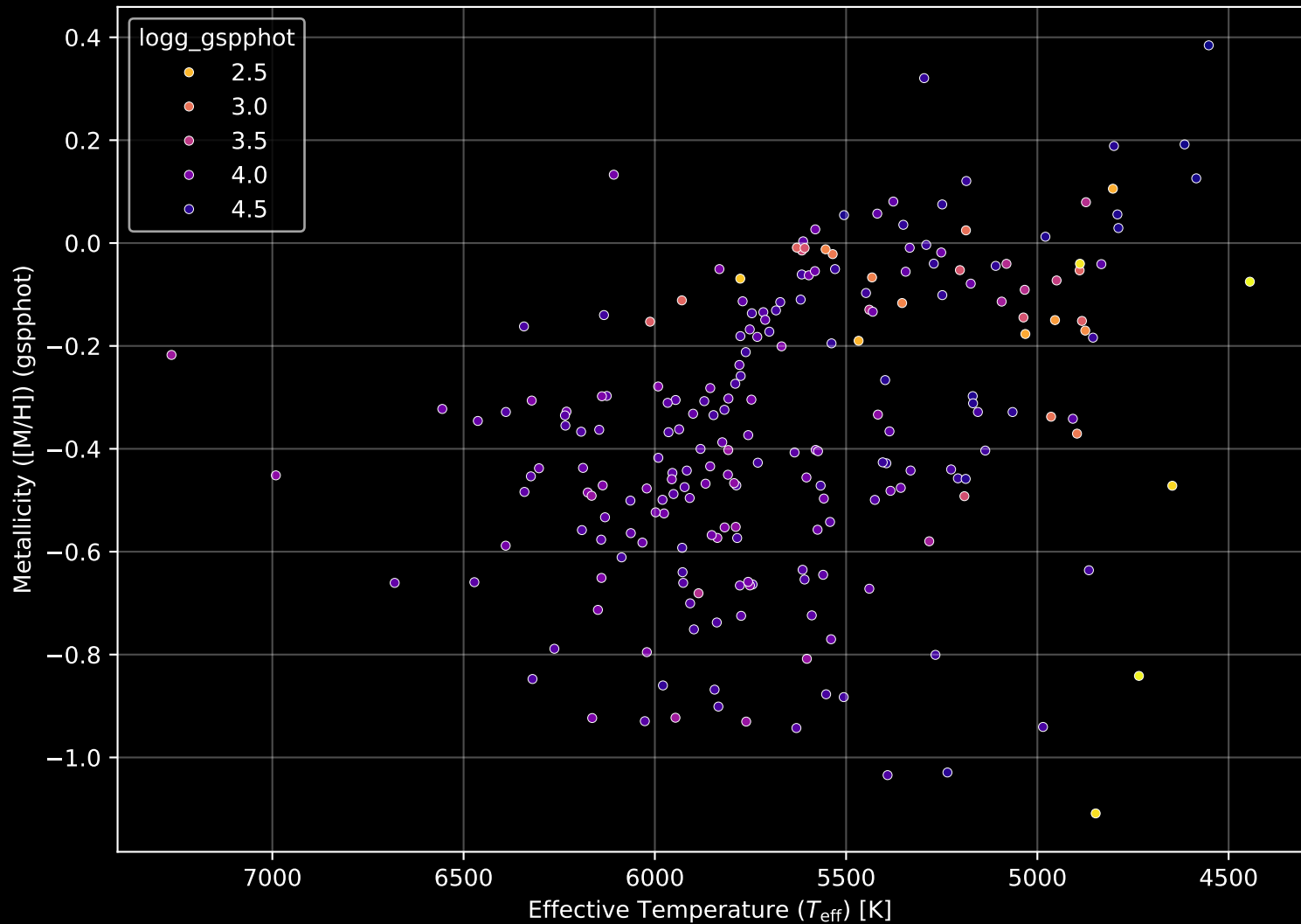
GALAH DR4 Field: [548] Stellar Population Parameters (n= 221)
