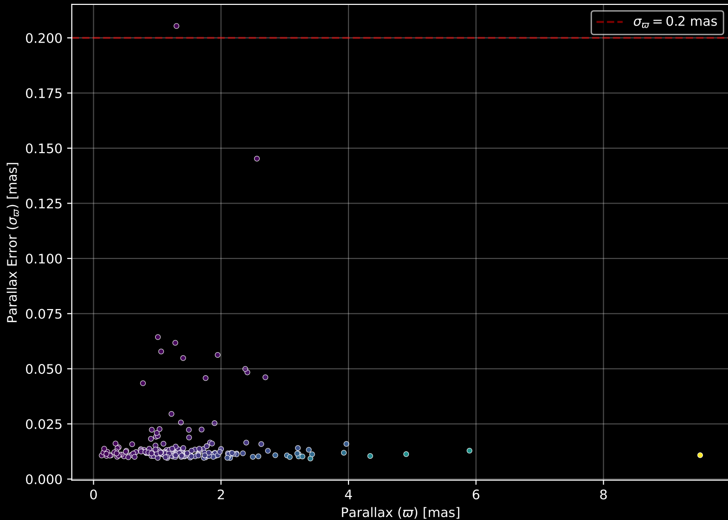
GALAH DR4 Field: [548] Parallax Quality (n= 221)
